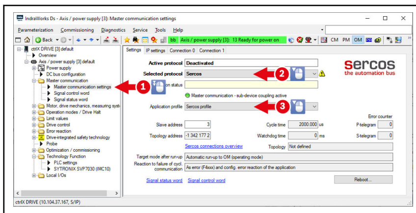
Fig. 7-16: Activate Sercos®
